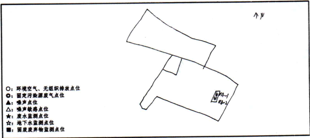
采样点位图
